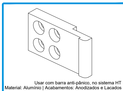
202334 CONTRA-FECHO HT P/ BARRA ANTI-PÂNICO
