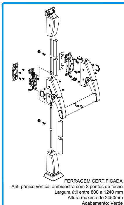
200991 ANTI-PÂNICO VERTICAL 6010.2/1200
