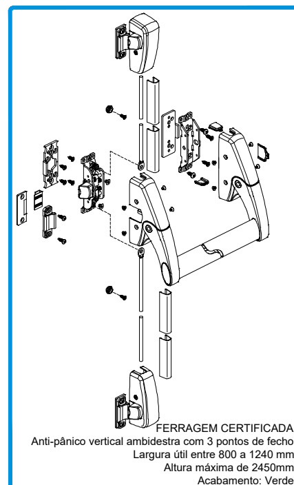
200992 ANTI-PÂNICO VERTICAL 6010.3/1200
