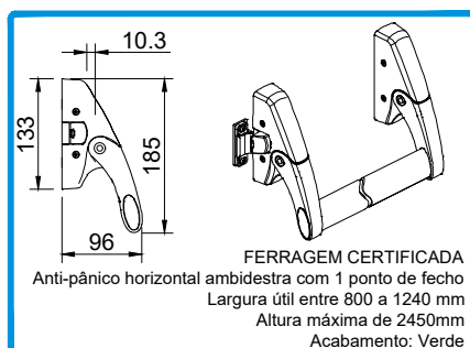
200993 ANTI-PÂNICO HORIZONTAL 6010.1/1200
