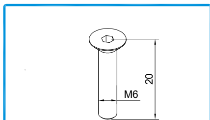
Para fixação do braço pivotante ao braço do motor Material: Inox | Acabamento: Inox 290128 PARAF. DIN7991 M6x20 INOX A2
