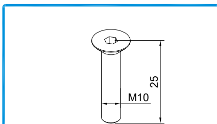
Para fixação do braço do motor ao perfil móvel inferior Material: Inox | Acabamento: Inox 290129 PARAF. DIN 7991 M10x25 INOX A2
