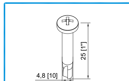
Para fixação do braço do motor ao perfil móvel inferior Material: Inox | Acabamento: Inox 290130 PARAF. AT/PF DIN7504-N 4,8x25 A2
