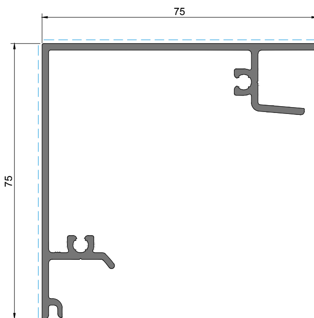
HT 22 Aro fixo Fixed frame | Cadre dormant
