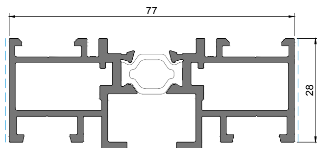
HT 22 Aro fixo Fixed frame | Cadre dormant
