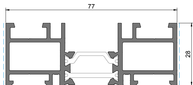
HT 02 Aro fixo Fixed frame | Cadre dormant
