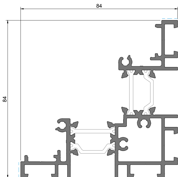
HT 55 Perfil de canto Corner profile | Profilé du coin
